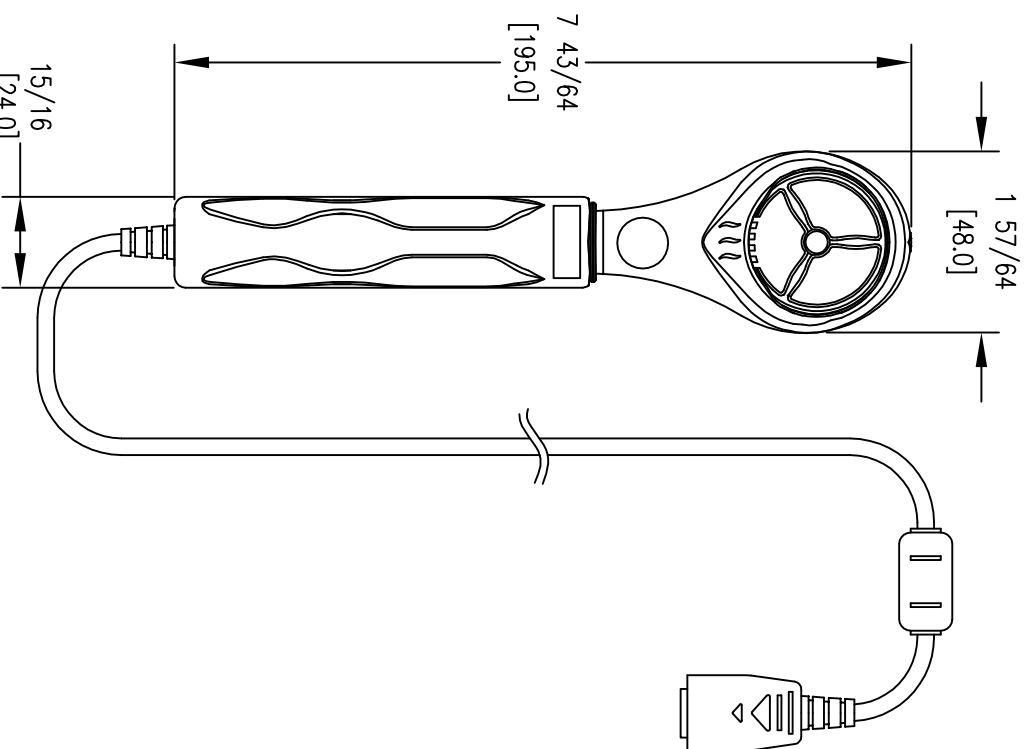
MINI VANE PROBE W/CABLE 35.4" (90 CM) LONG
